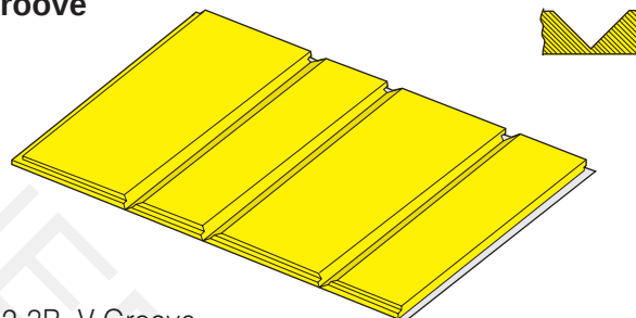
Fig. 2-3B. V-Groove.
